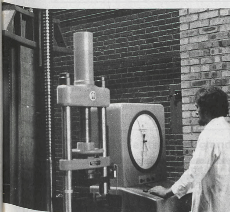
Essai de résistance à la compression sur une brique de hauteur d'étage
